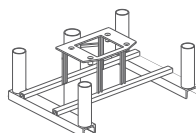
Universalrahmen OPI2020 für Betonguss E-No 39.00113.00
